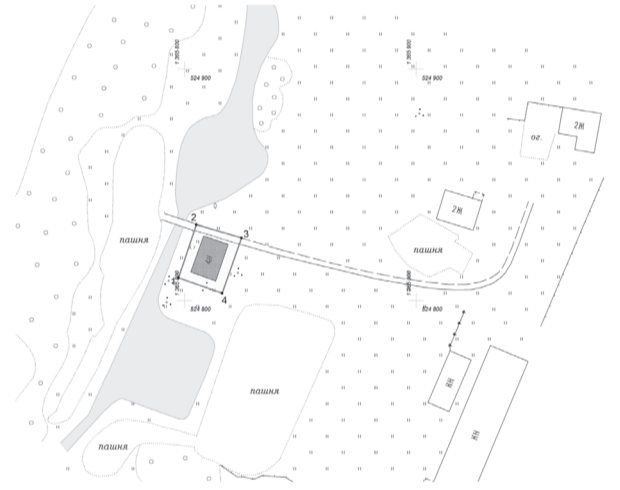
3. Схема границы территории
